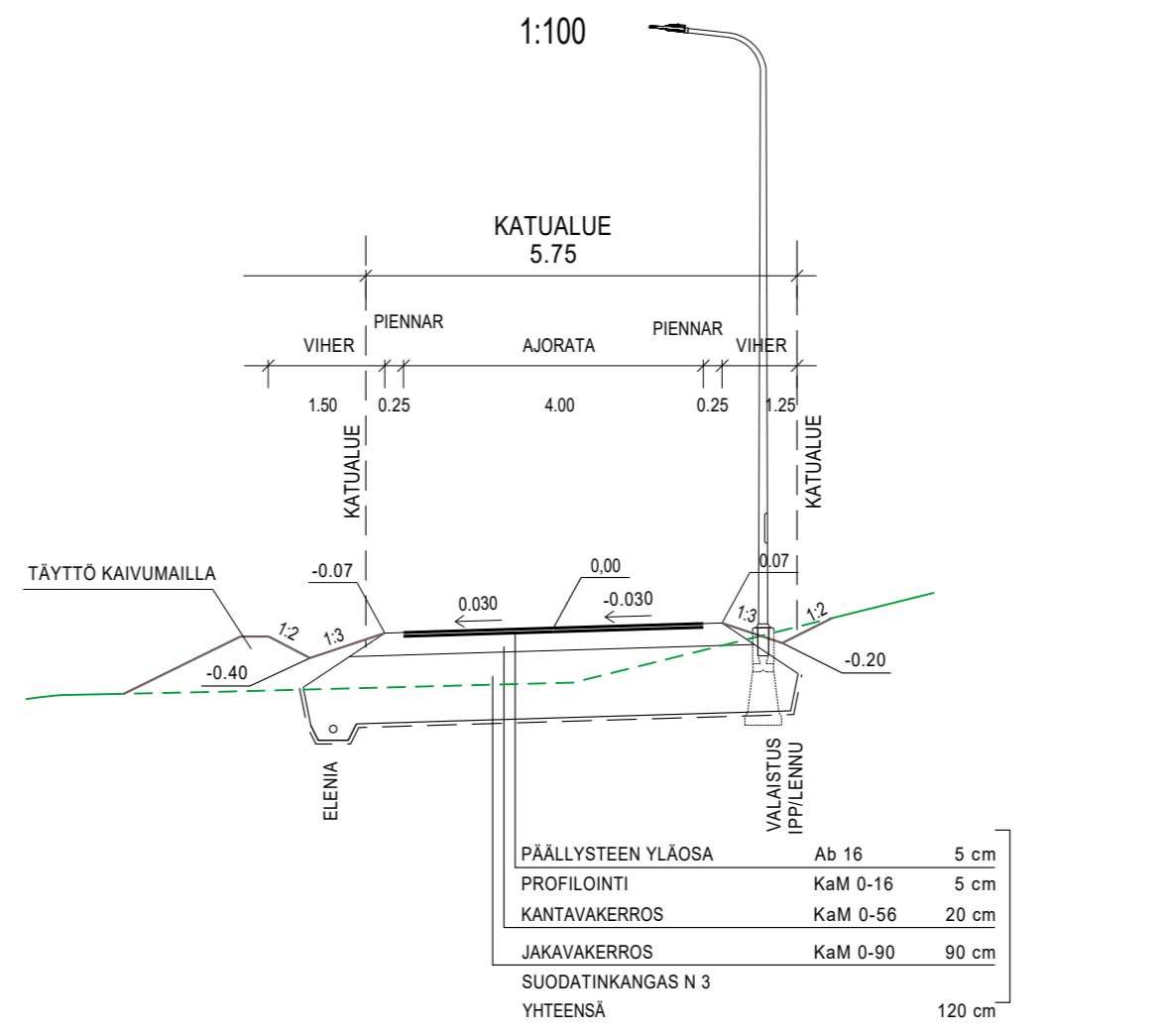
TYYPPIPOIKKILEIKKAUS PAALULTA 400
