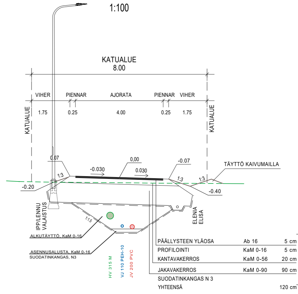
TYYPPIPOIKKILEIKKAUS PAALULTA 220
